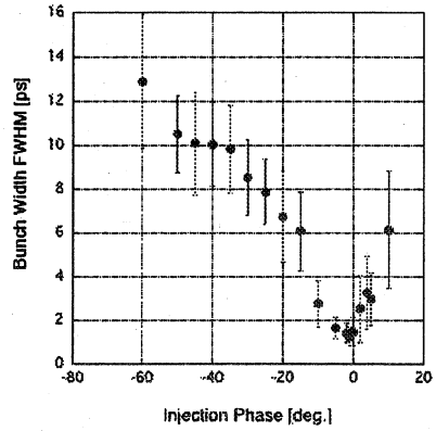
図3 加速管入射位相に対するバンチ幅 (FWHM)
