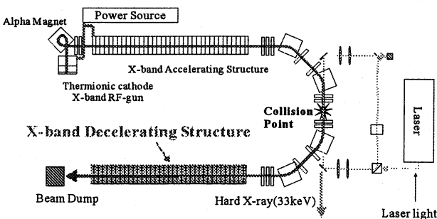
図5 減速管を導入した X バンド体系図
