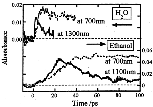
図2 Mg photocathode RF gun で測定した、水およびエタノール電子の溶媒和過程
