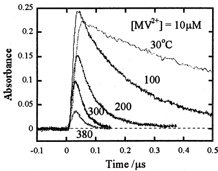
図1 高温・超臨界水中の水和電子とメチルビオローゲンとの反応
