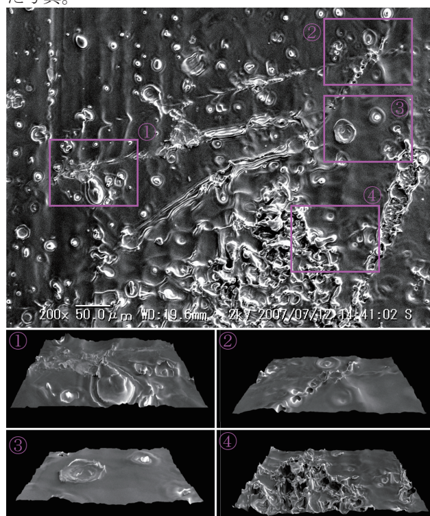
図7：SEMによる3D表面観察例。
