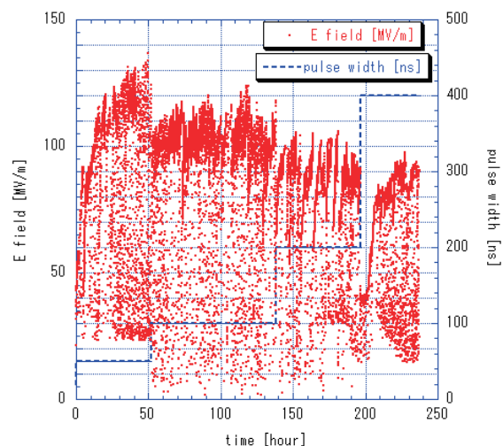
図4：Cu-002狭導波管RFプロセッシング履歴、電界強度とパルス幅。
