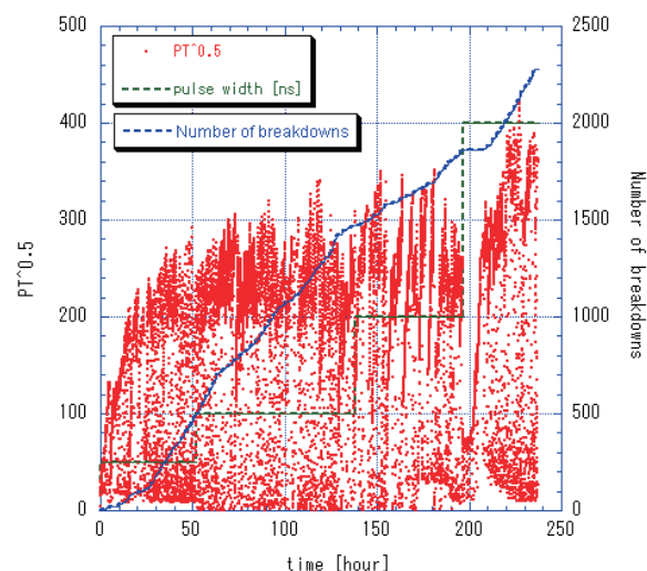
図5：Cu-002狭導波管RFプロセッシング履歴、P*T 1/2 値と放電頻度及びパルス幅。
