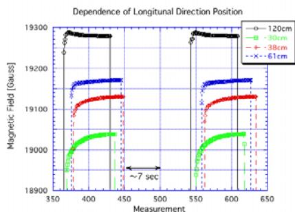
図1 偏向電磁石の磁場変化の位置依存
