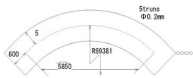
図2 ピックアップコイル外形
