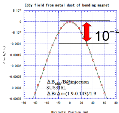
図3 真空ダクトの渦電流による磁場の歪み (2001/11/16第二回大強度陽子加速器計画技術報告会、湯浅由将氏による)
