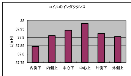
図7 コイルのインダクタンス
