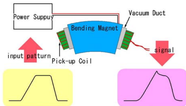
図8 ピックアップコイルを含む測定系
