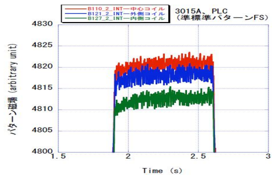
図10 偏向電磁石磁場変化
