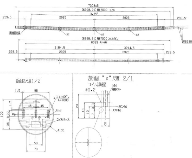
図4 測定装置全体図
