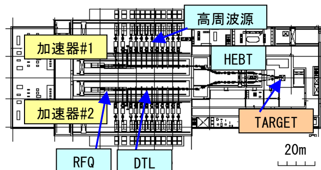
図1 : IFMIF 加速器システムのレイアウト
