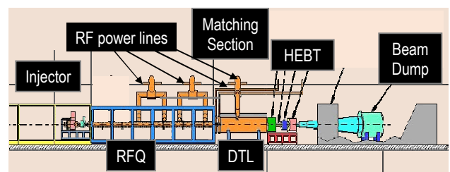
図3：プロトタイプ加速器の構成
