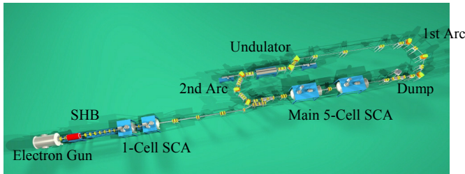
図2：JAEA-ERLの概略図
