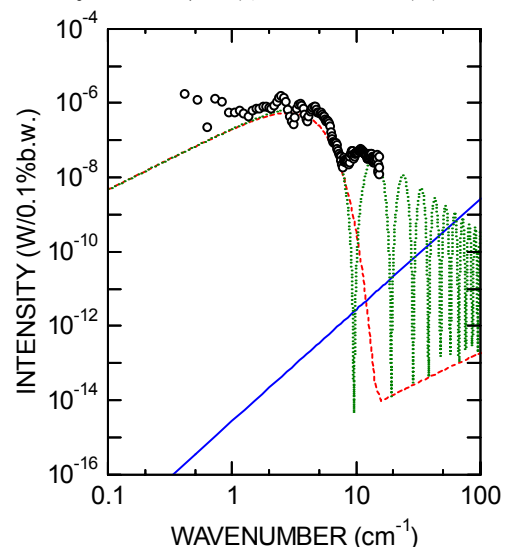
図4：観測されたCSRスペクトル（丸印）。実線は高圧水銀灯のスペクトル強度。破線は4 psのガウス分布のバンチ、点線は3.5 ps(FWHM)の三角形のバンチを仮定した場合の計算値。
