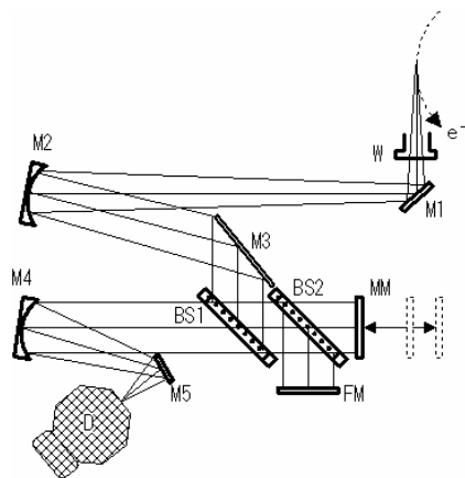
図3：実験装置の模式図。W: 真空窓、M1, M3, M5: 平面鏡、M2: 球面鏡(f1500)、M4: 球面鏡(f410)、FM: 固定鏡、MM: 移動鏡、BS1, BS2: ビームスプリッター、D: Siボロメータ
