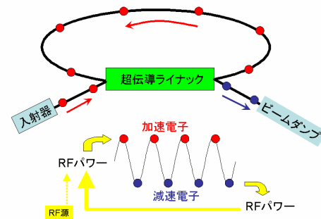
図1: ERLの原理を示す模式図
