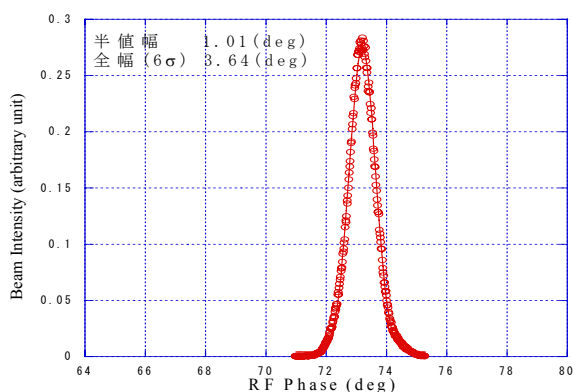
図4 : Ne260MeVのビーム位相分布
